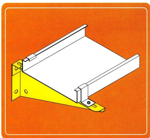
三角型壁架 3-BRACKEETS
