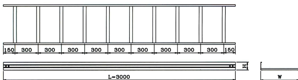
邊槽高度 80H 系列 (80mm HEIGHT SERIES)
